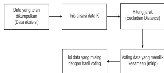
Gambar 2. Tahapan data preprocessing dengan KNNImputer
