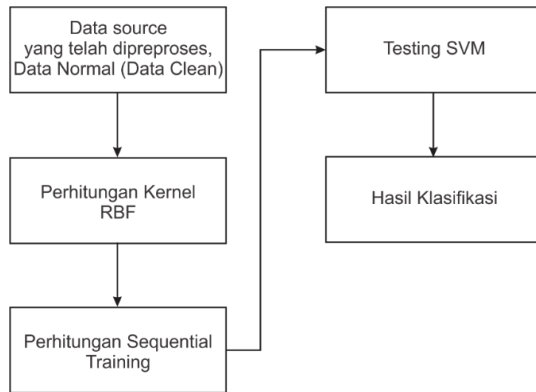
Gambar 3. Tahapan Pemodelan dengan SVM
