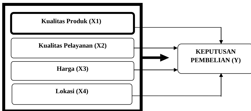
Gambar 1. Kerangka Konseptual
